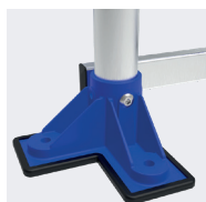
Pieds double fixation. Vis Ø 8 mm (non fournie, type à choisir en fonction du sol)
