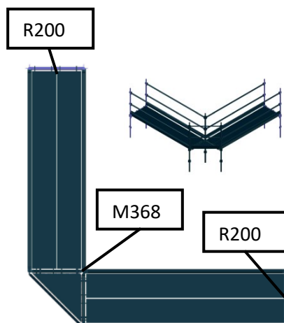
Figure 68 - Angle à 3 poteaux avec plateau d'angle en extérieur
