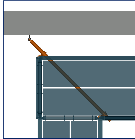
Figure 50: Amarrage dans un angle (vue de dessus)
