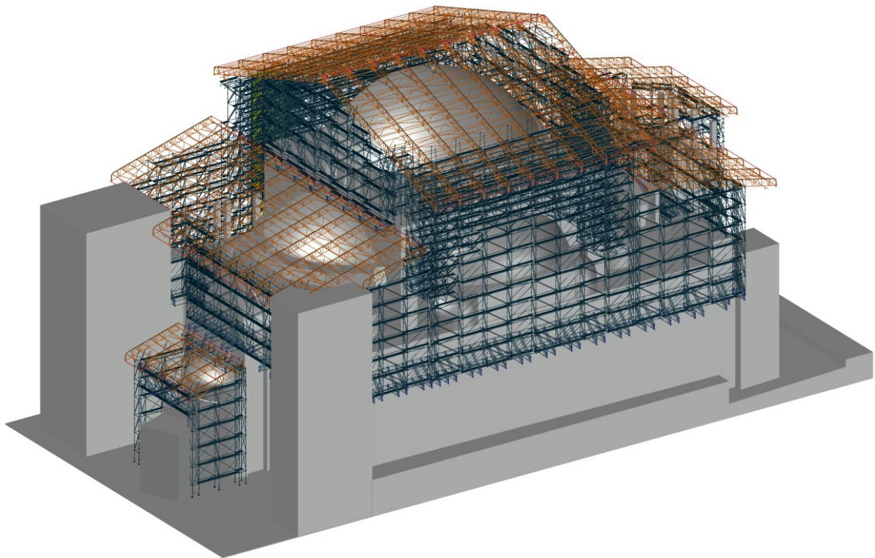
Figure 87 : Exemple d'un échafaudage équipé d'un parapluie
