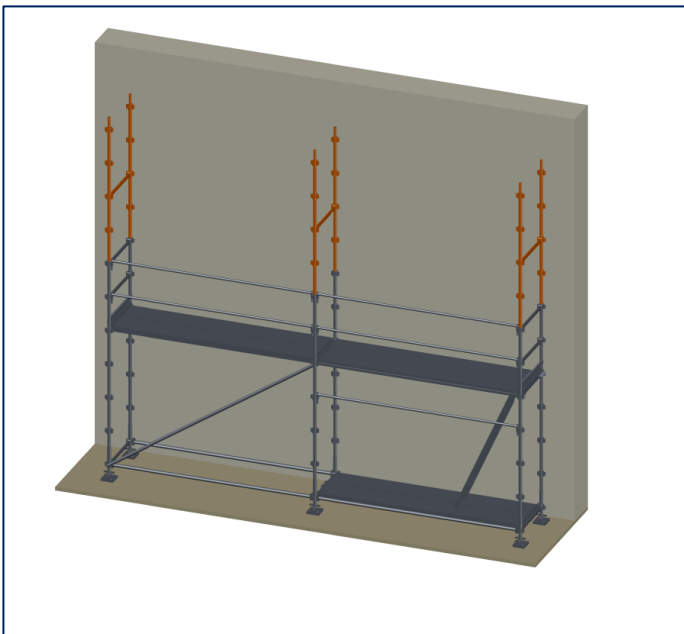
Étape 11 : Ajouter les montants et les longerons pour le niveau d'après. Goupiller par RCM12.
