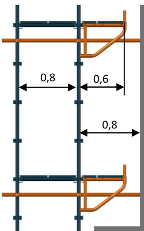
5 – Console de 0,6m
