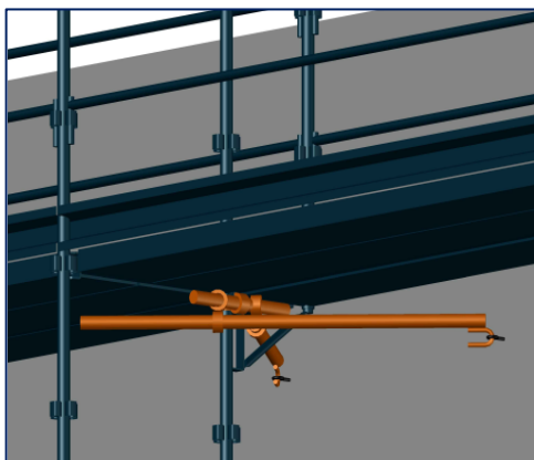
Figure 47 : Amarrage en V avec console de 0,40 m
