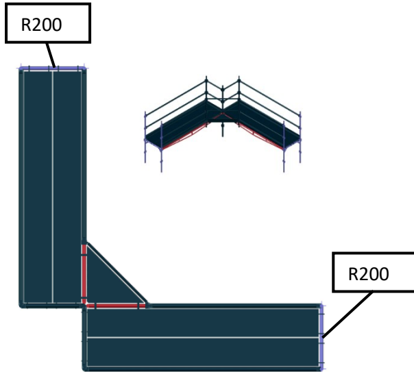
Figure 70 - Angle à 3 poteaux avec plateau d'angle en intérieur
