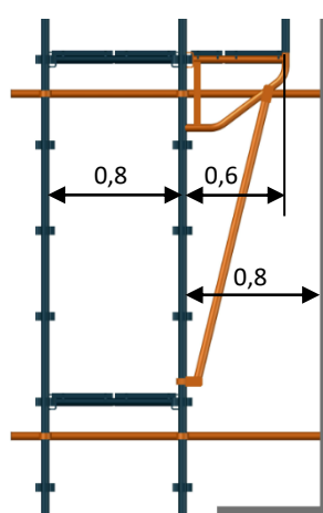
6 – Console de 0,6m
