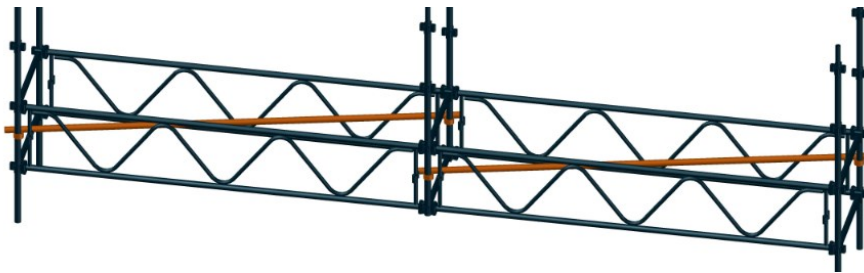
Figure 83 : Laçage sur poutre acier
