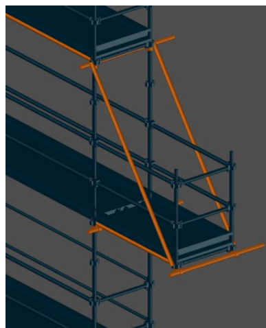
10 – Déport supérieur à 1m
