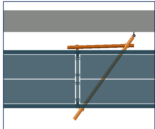
Figure 46 : Amarrage déporté (vue de dessus)
