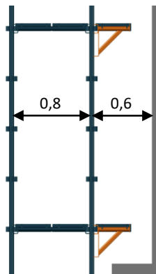
2 – Console de 0,4m sans manchon
