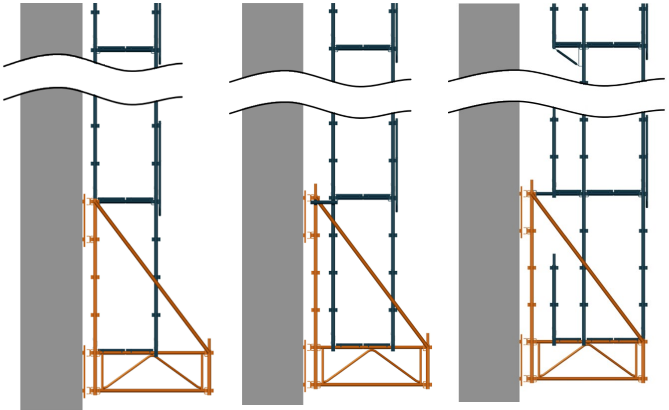
3 – Échafaudage simple piquage avec console de 0,40m en intérieur
