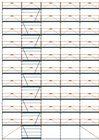
Figure 30 : Diagonalisation avec Fusio (type DV ou RCM)
