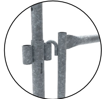
Figure 23 : Assemblage crochet Fusio
