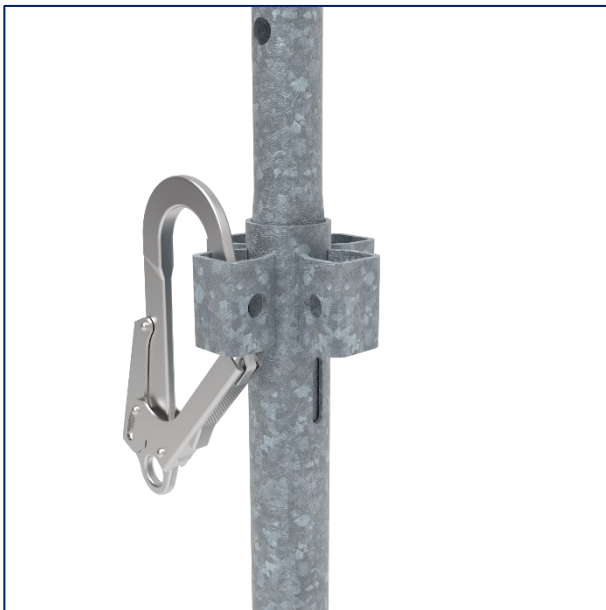
Figure 14 : Point d'accroche sur le nœud M368 d'un poteau à 1 m au-dessus du plancher sur lequel se trouve le personnel
