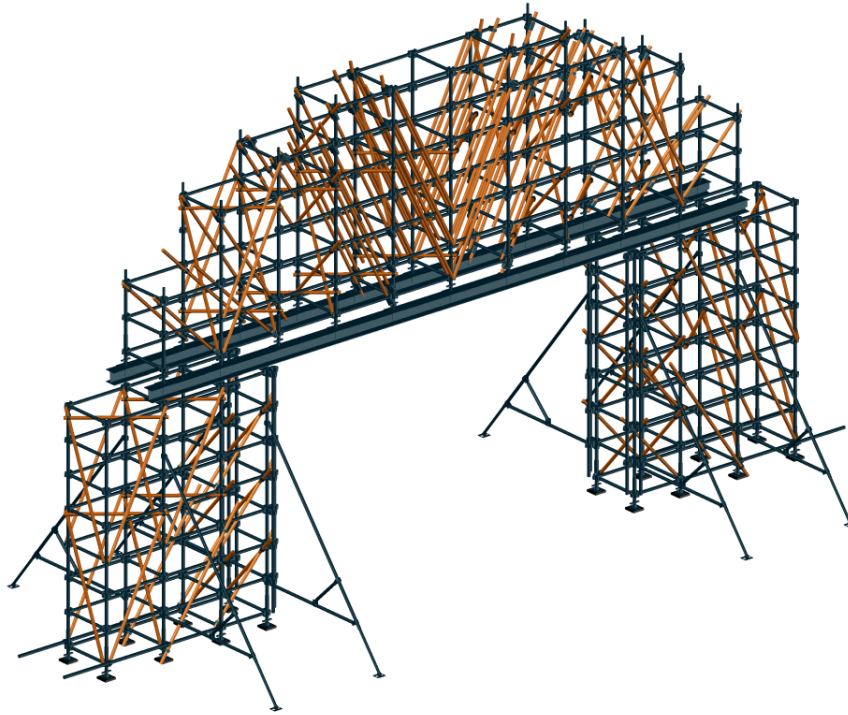
Figure 35: Cas de diagonalisation complexe
