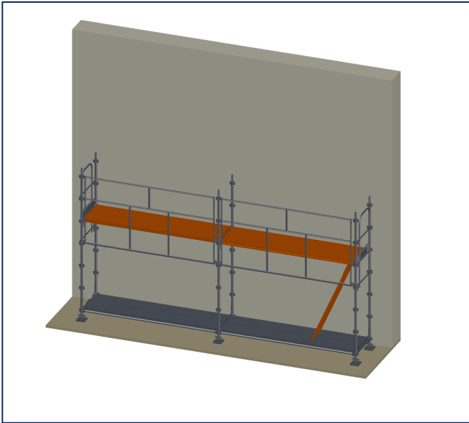
Étape 8 : Ajouter les planchers du niveau supérieur.
