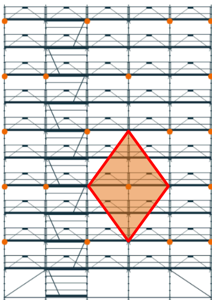
Figure 38 : Cas 1 – Échafaudage non recouvert
