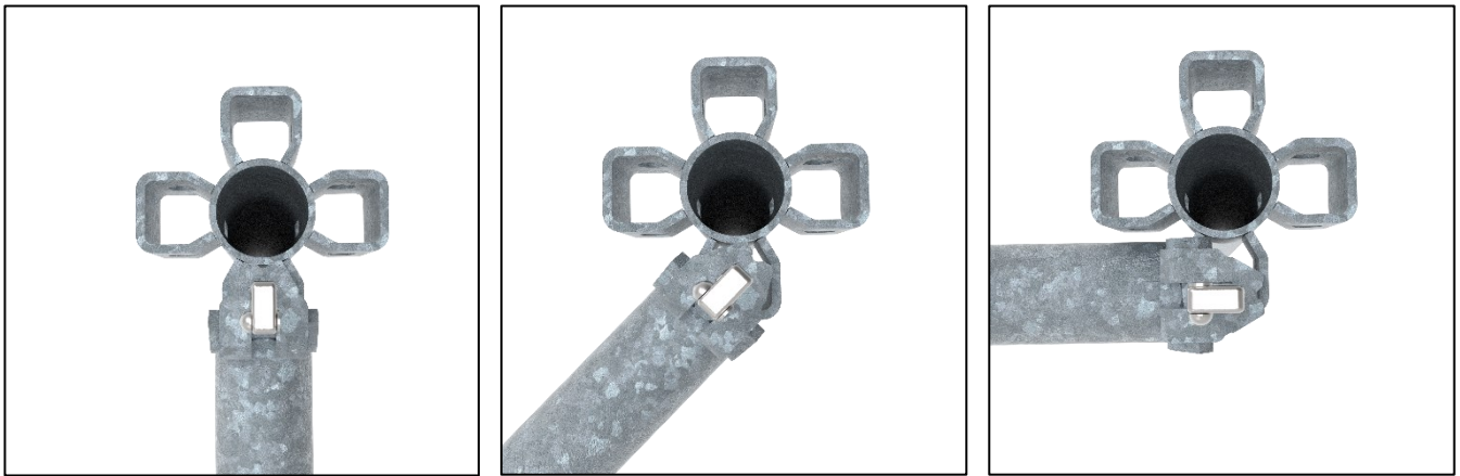
Figure 4: Montage à 0° (gauche), 45° (centre) et 90° (droite) d'un longeron sur le nœud M368
