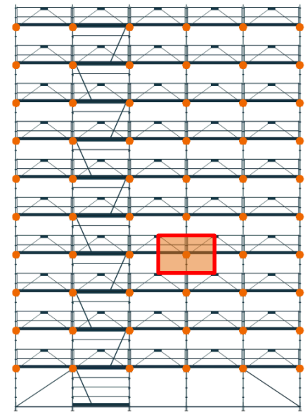
Figure 38: Cas 3 – Échafaudage recouvert d'une bâche
