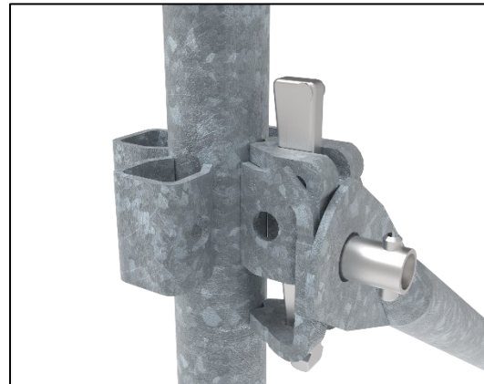
Figure 6 : Nœud M368 avec diagonale type RCM
