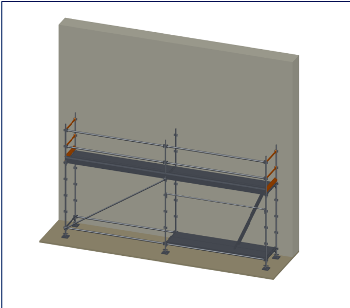
Étape 9 : Monter les GC d'extrémité.
