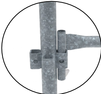
Figure 24 : Assemblage lisse sur douille carrée
