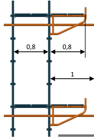
7 – Console de 0,8m
