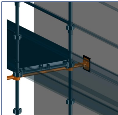
Figure 55 : Butonnage 3D
