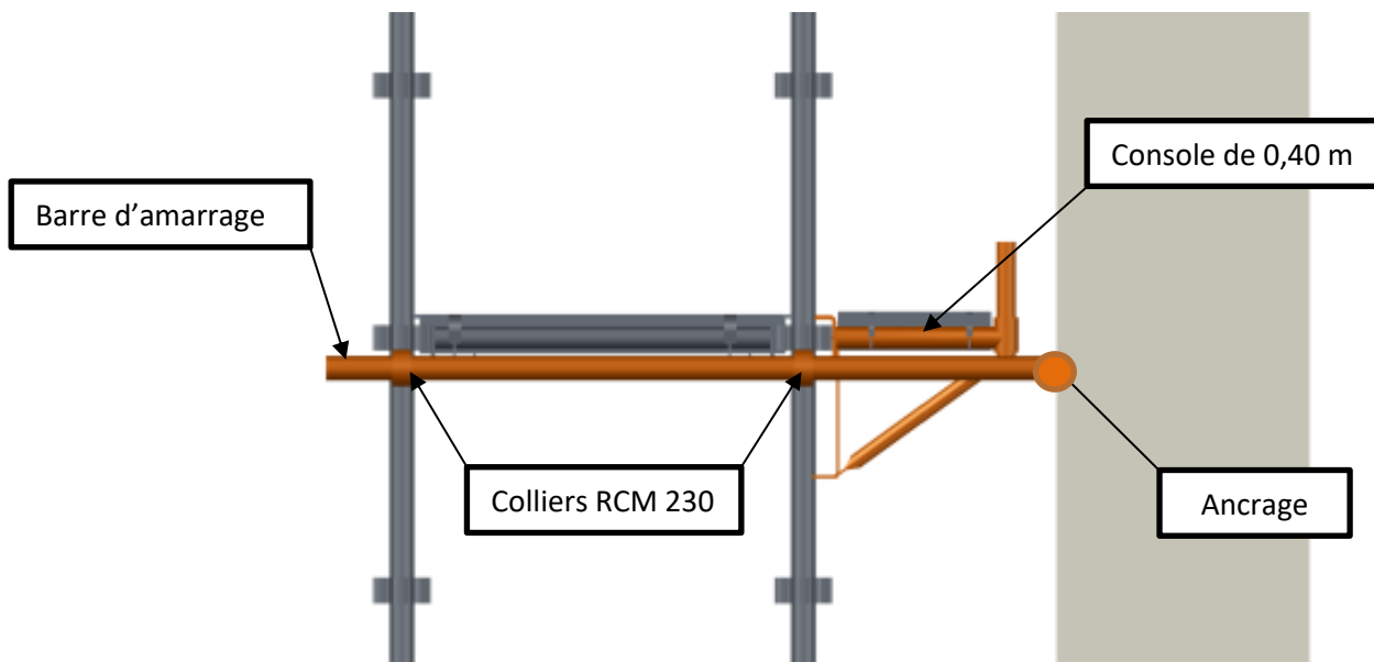
Figure 75: Exemple d'une console 0,40 m sur file intérieure
