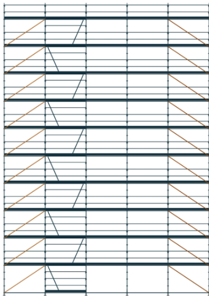
Figure 28 - Diagonalisation avec lisses ou longerons (type DV)
