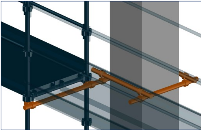
Figure 58 : Ceinturage 3D
