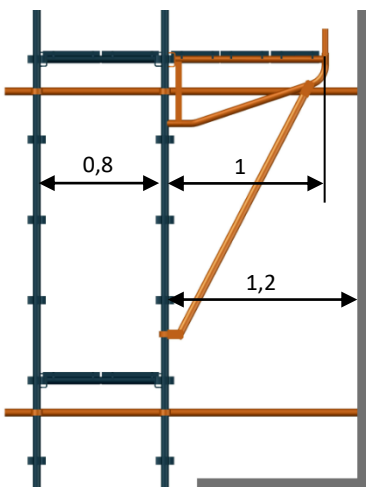
9 – Console de 1m
