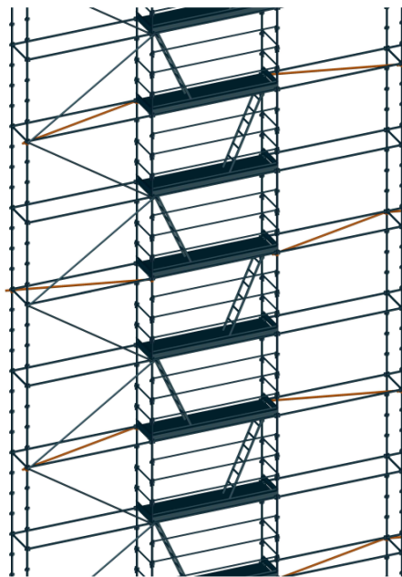
Figure 34 : Exemple de diagonalisation horizontale
