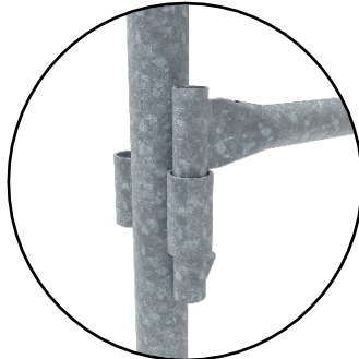
Figure 22 : Assemblage lisse sur douille ronde
