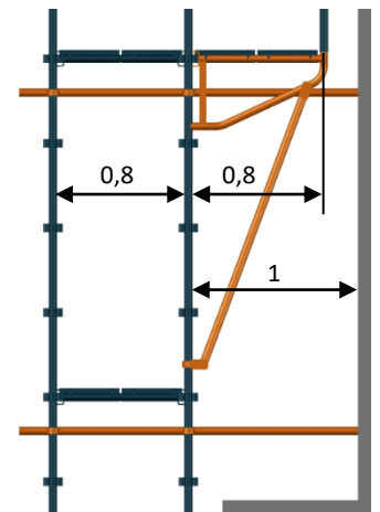
8 – Console de 0,8m
