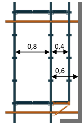
4 – Console de 0,4m avec manchon
