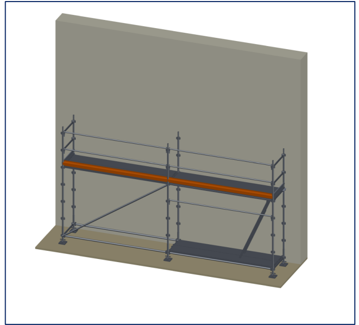
Étape 10 : Ajouter les plinthes pour sécuriser le niveau.
