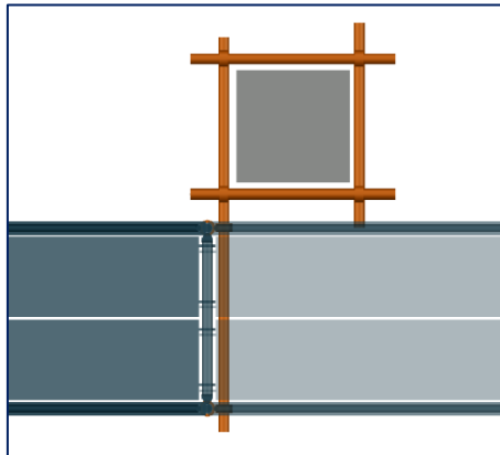
Figure 60: Ceinturage (vue de dessus)
