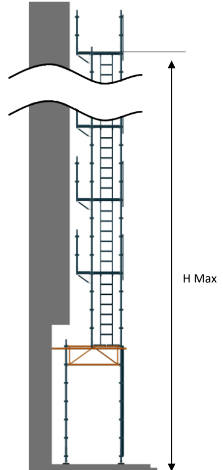
Figure 81: Passage piéton poteau extérieur
