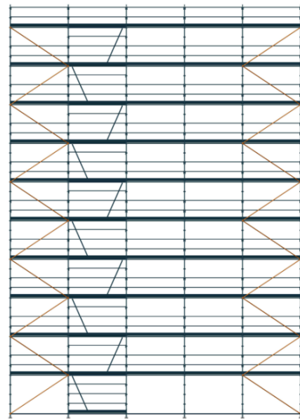
Figure 29 - Diagonalisation avec lisses ou longerons (type RCM)
