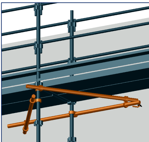
Figure 41 : Amarrage en V sur file extérieure
