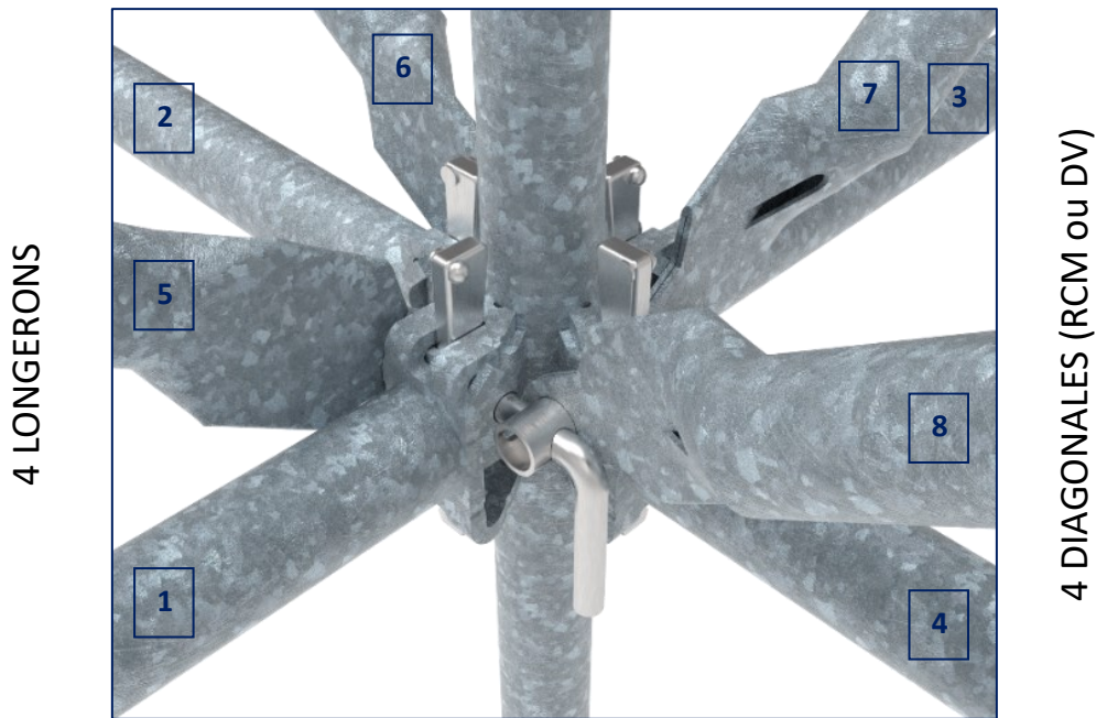
Figure 2 : Nœud M368 avec 8 positions d'éléments
