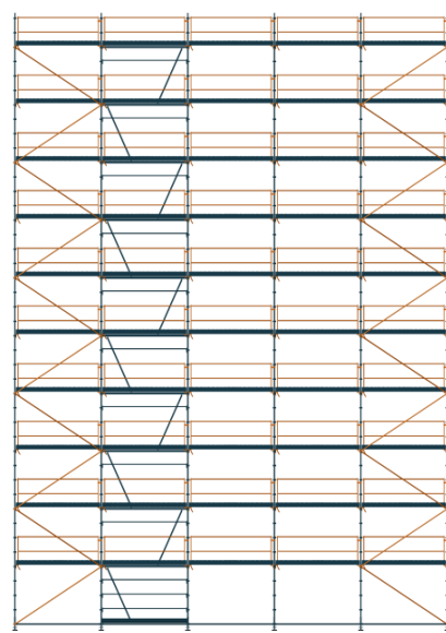
Figure 31 : Diagonalisation avec SecuritUp (seulement RCM)
