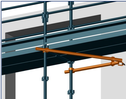
Figure 45 : Amarrage déporté
