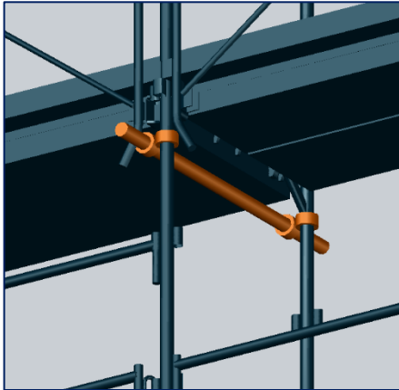
Figure 39 : Amarrage en ligne
