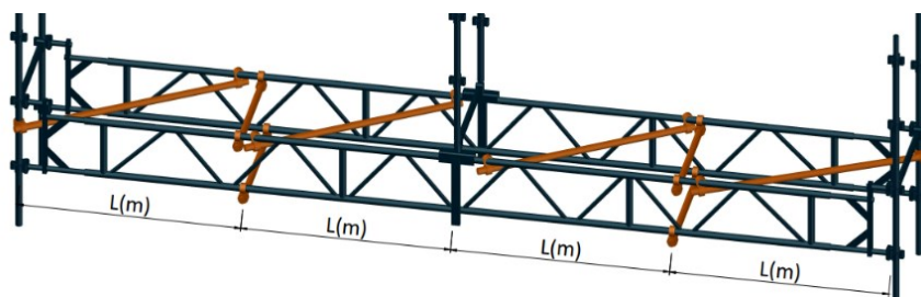
Figure 84 : Laçage sur poutre alu (longueur L à déterminer suivant le moment admissible des poutres)
