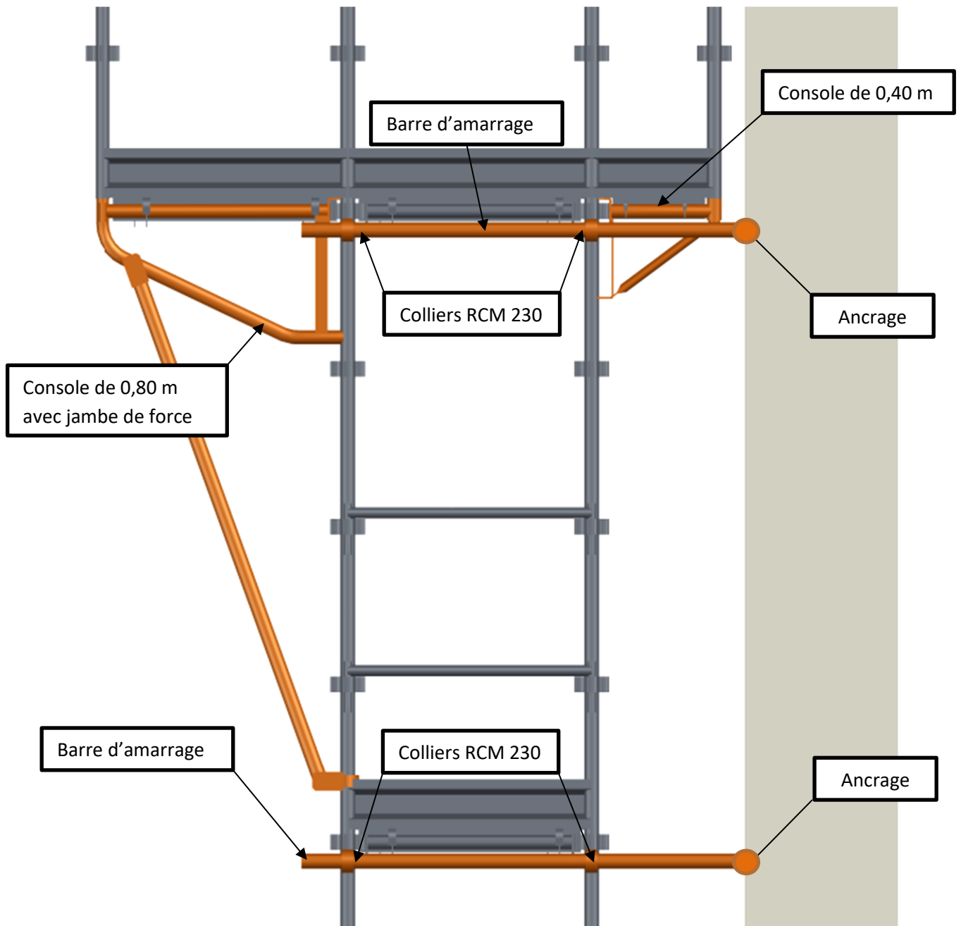
Figure 77 : Exemple de consoles placées au dernier niveau
