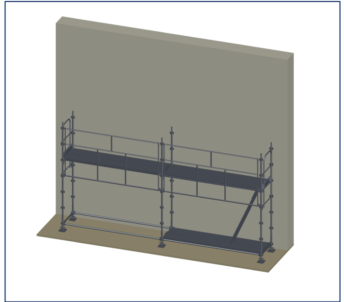
Les GC et planchers étant installés, accéder au niveau supérieur. Faire hisser les éléments (longerons ou lisses) depuis le sol par un autre opérateur.
