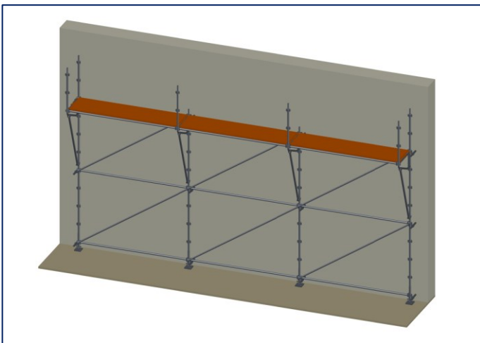
Étape 7 : Mettre en place les planchers.
