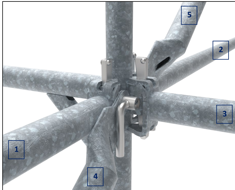
Figure 7 : Nœud R200 Progress avec 5 positions différentes
