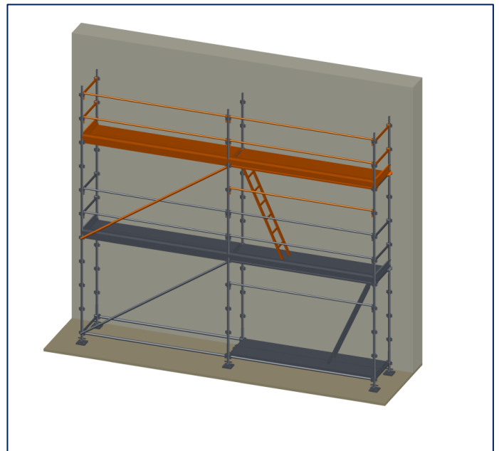
Étape 12 : Répéter les étapes de 5 à 11. Amarrer la structure depuis les niveaux inférieurs.
