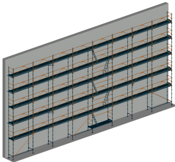
Figure 33: Exemple de contreventement vertical pour GC Fusio
