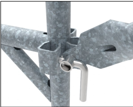
Figure 11 : Noeud R200 Progress avec diagonale type DV
