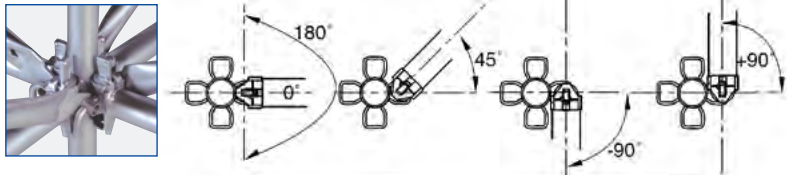
Possibilité de montage à 180° sur chaque douille. Seul le montage à 0° autorise les porte-à-faux.
