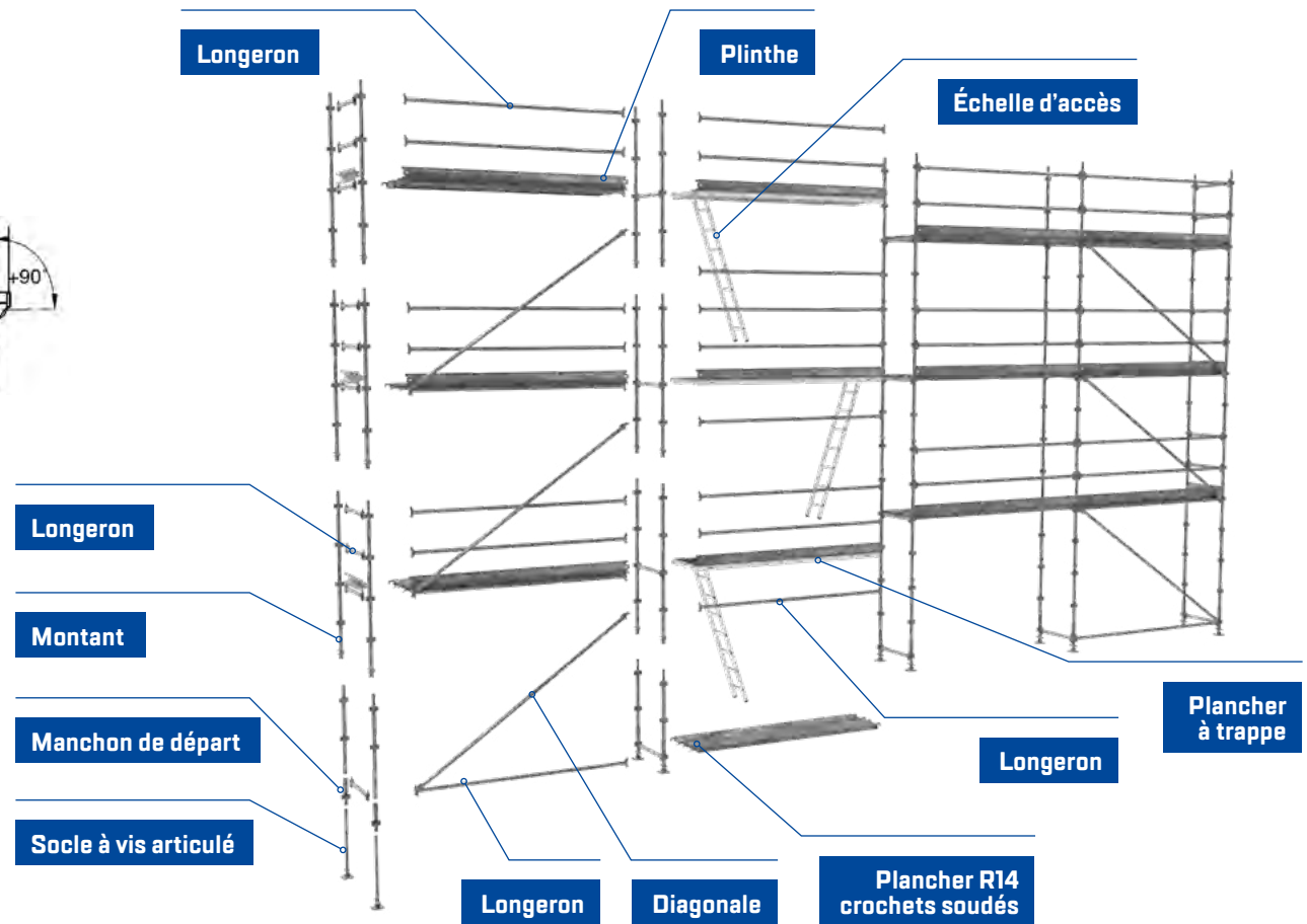
Schéma de principe
