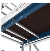
Plancher alu-bois à poutre rapportées
