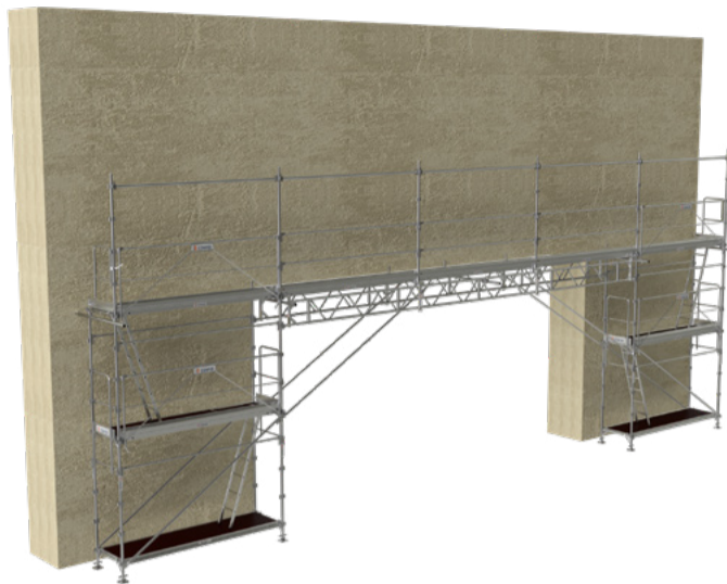
A Pont 6 m : 2 poutres aluminium de 5,10 m en vis à vis
